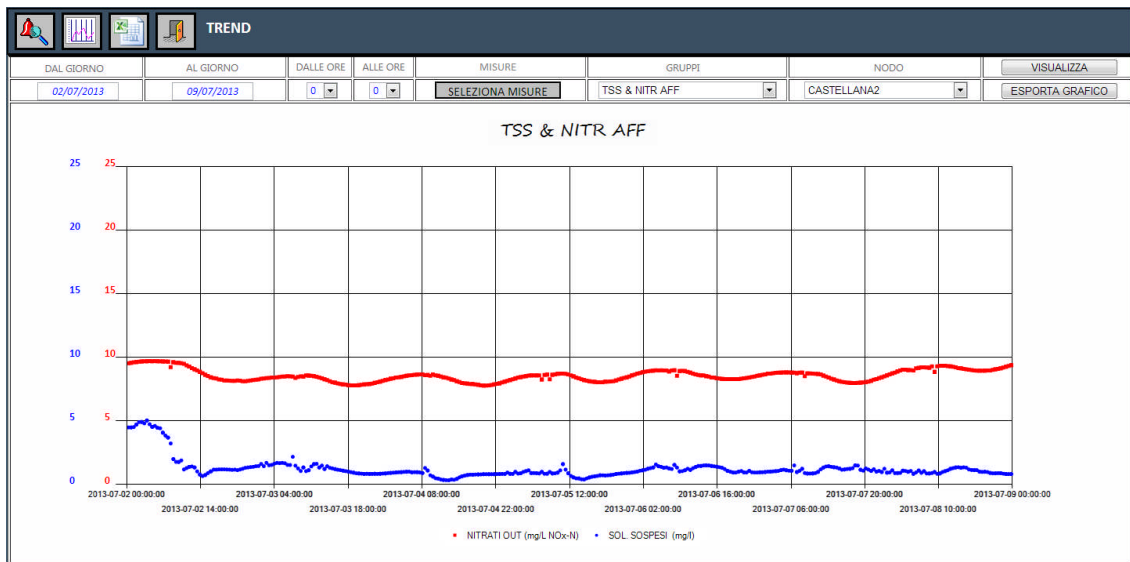
Figura 5 – Trend misure
