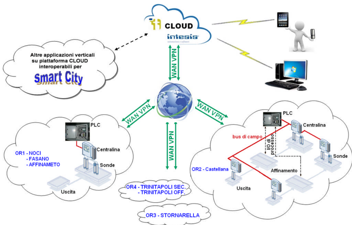
Figura 2 – Architettura del sistema: dal campo al Cloud
