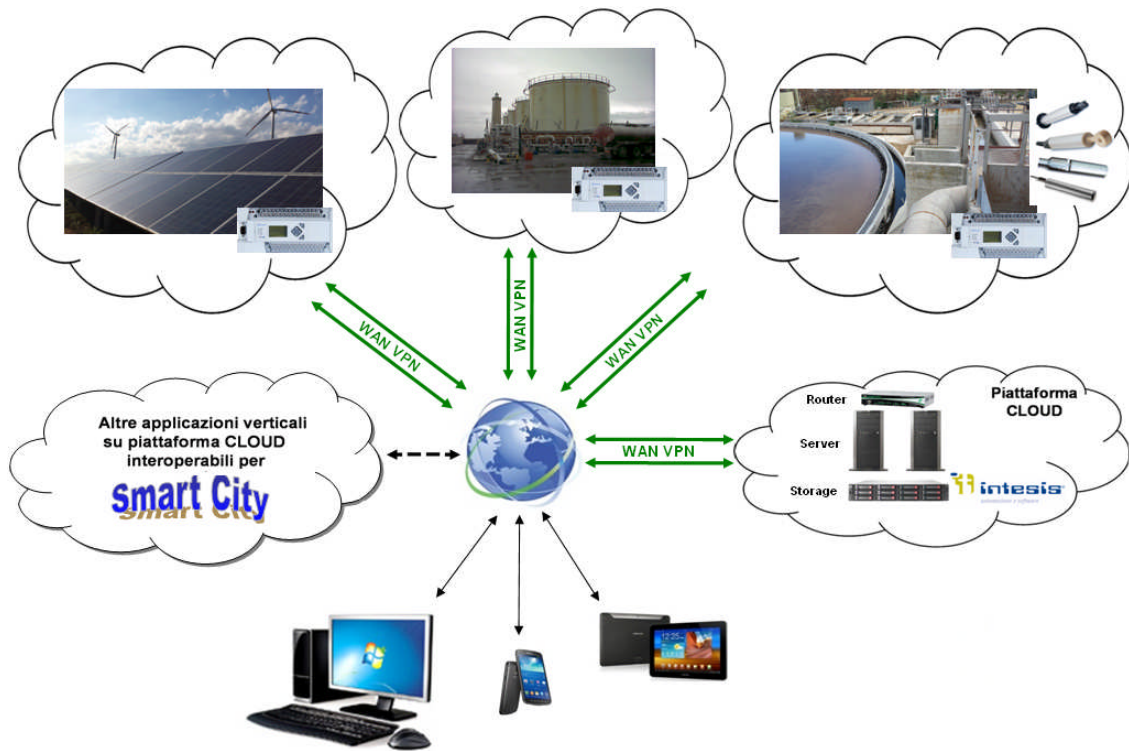
Figura 8 – Architettura di Cloud Computing per Smart Systems.
