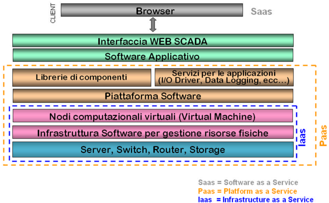
Figura 3 – La piattaforma di Cloud Computing
