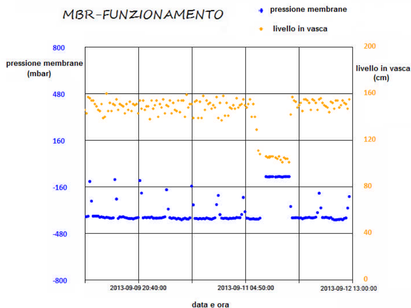
Figura 7 - TMP (TransMembrane Pressure) e livello in vasca in un impianto MBR.
